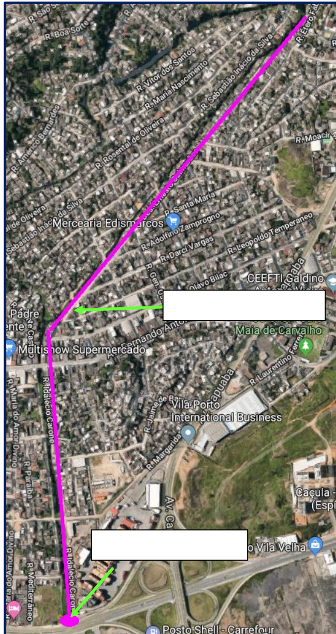
FIGURA 11 – LINHA DE RECALQUE EBAP ARIBIRI
