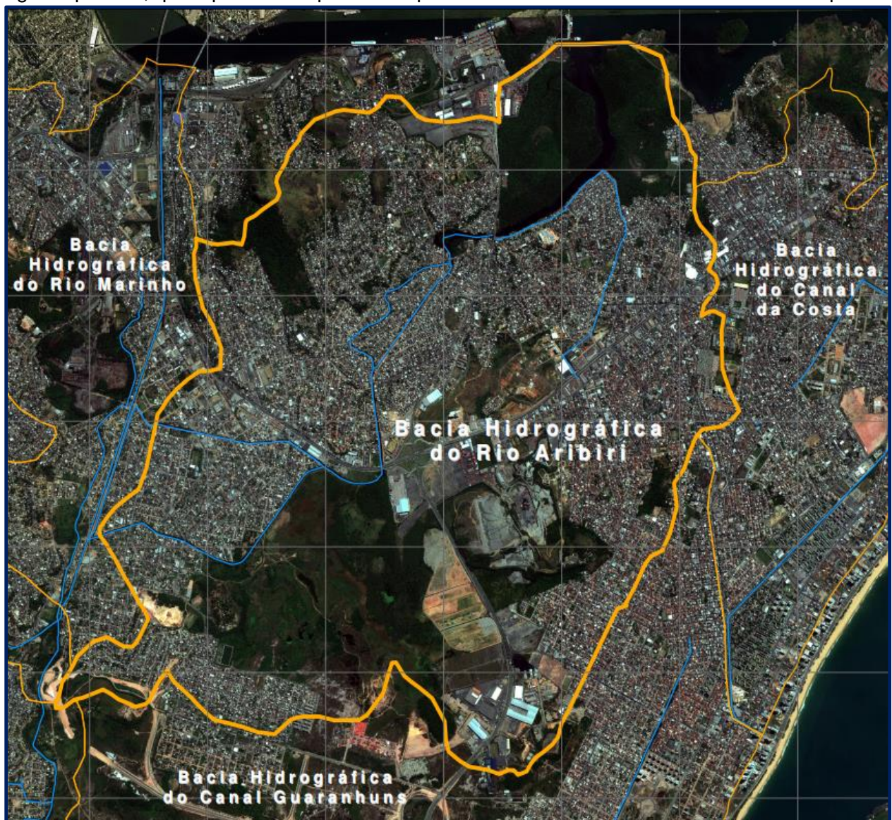
FIGURA 01 – IDENTIFICAÇÃO DA BACIA HIDROGRÁFICA DO RIO ARIBIRI
