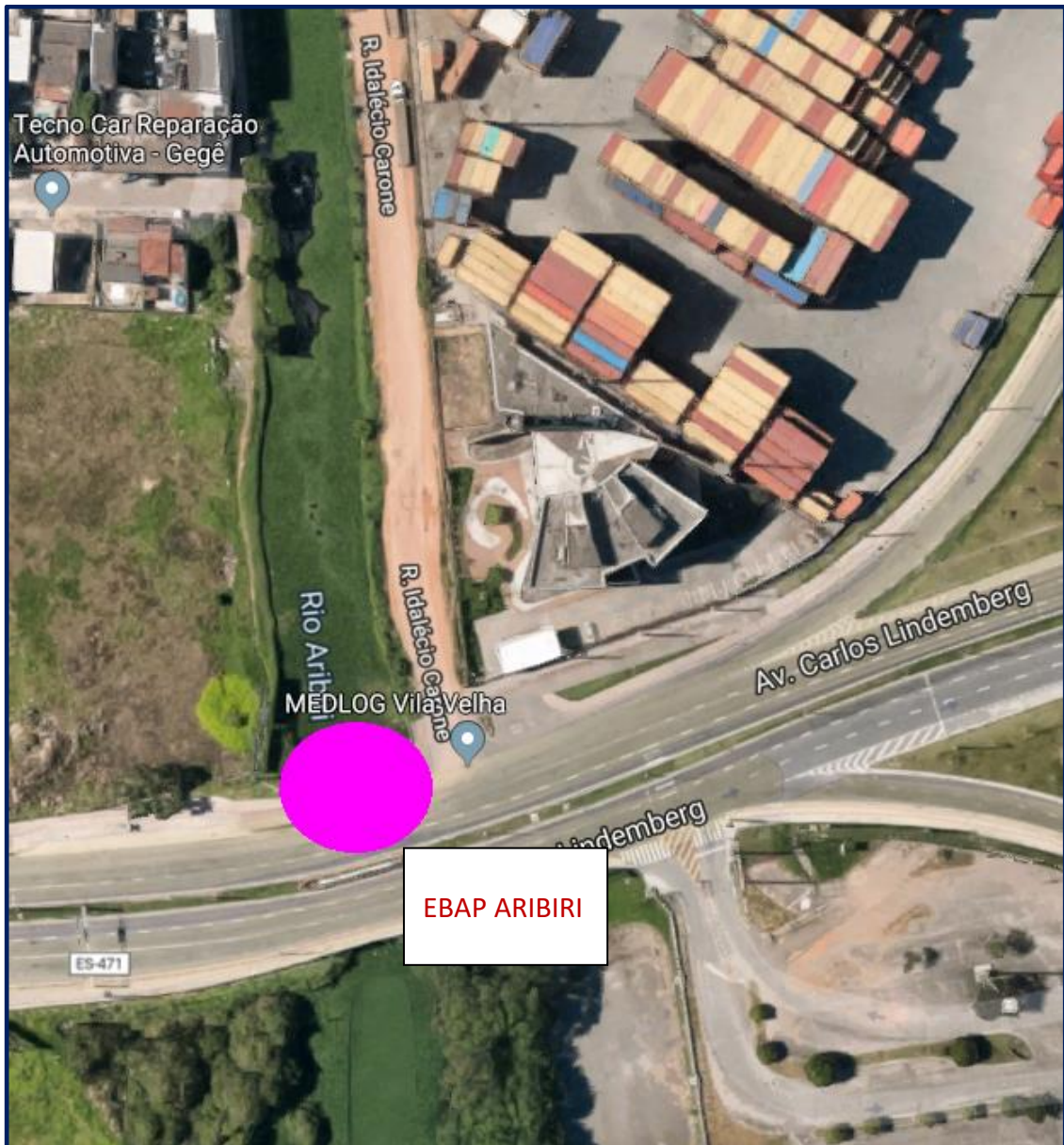
FIGURA 03 – LOCALIZAÇÃO EBAP ARIBIRI
