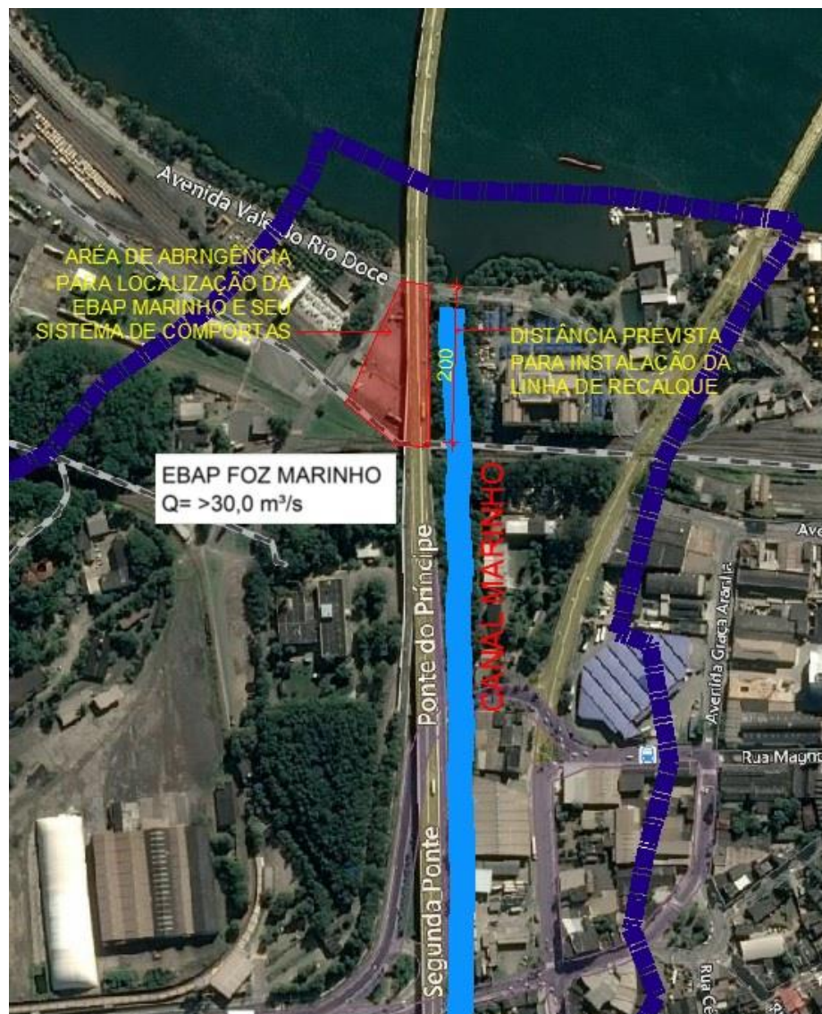
Figura 04 – Identificação das intervenções do Marinho: EBAP, Sistema de Comporta e Linhas de Recalque
