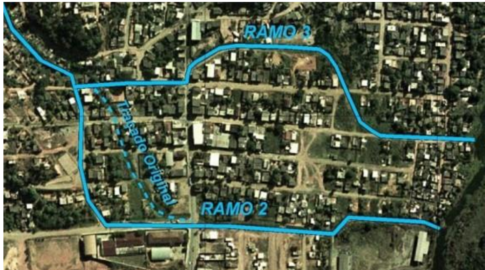
Figura 18 – Galeria e Dique Canal Marilândia
