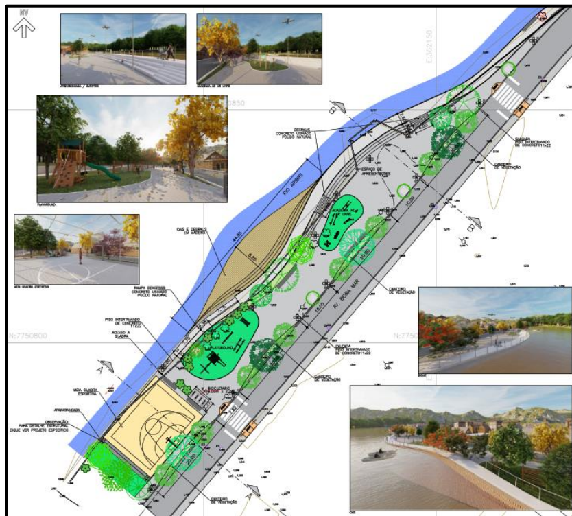
Figura 4 - Detalhes Dique Dom João Batista
