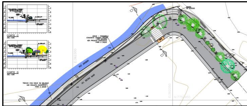
Figura 2 - Detalhes Dique Dom João Batista
