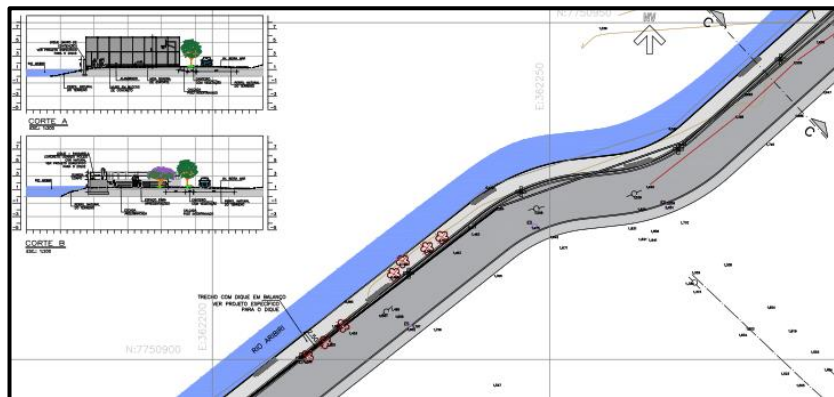
Figura 3 - Detalhes Dique Dom João Batista
