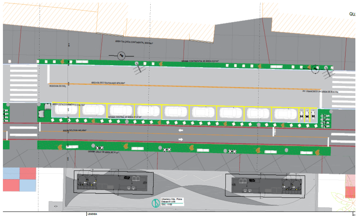
Figura 2 - Detalhes obra de urbanização
