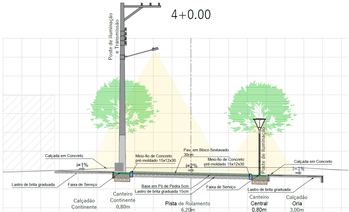
Figura 6 - Detalhes obra de urbanização
