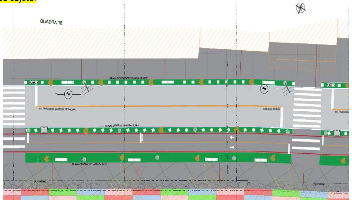
Figura 3 - Detalhes obra de urbanização
