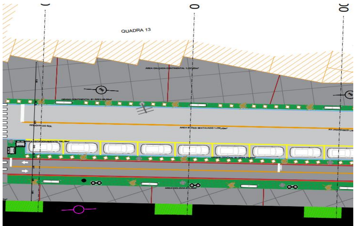
Figura 1 - Detalhes obra de urbanização
