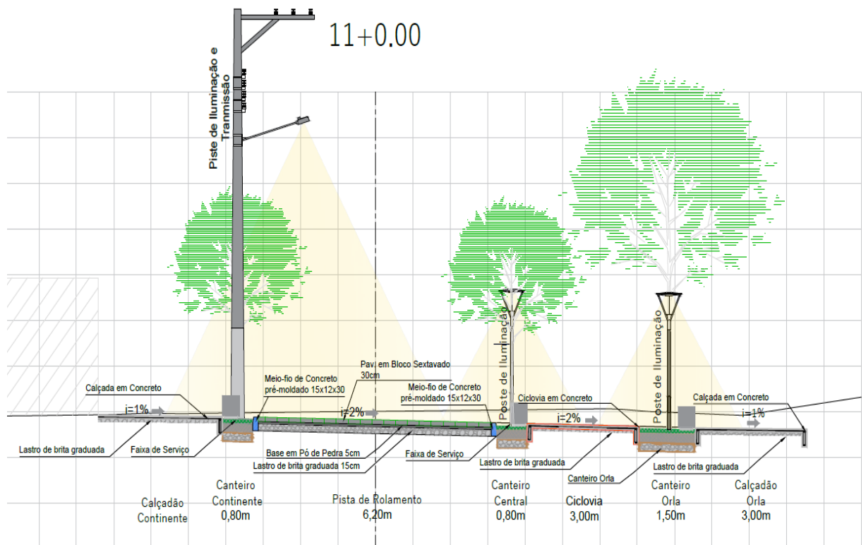
Figura 5 - Detalhes obra de urbanização
