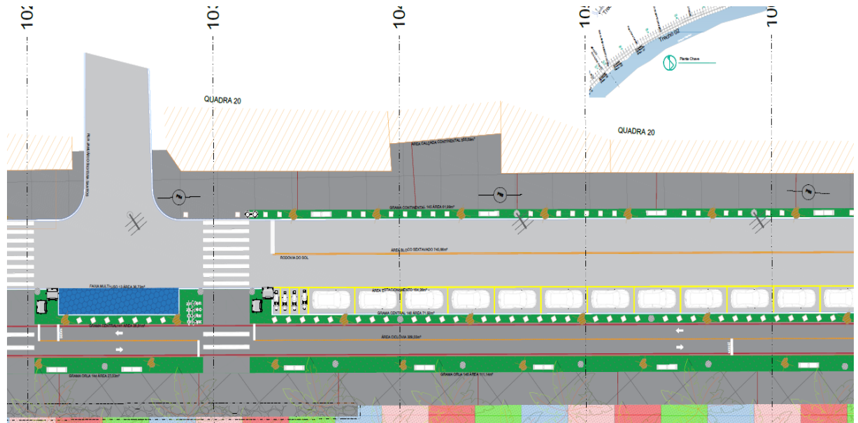
Figura 4 - Detalhes obra de urbanização
